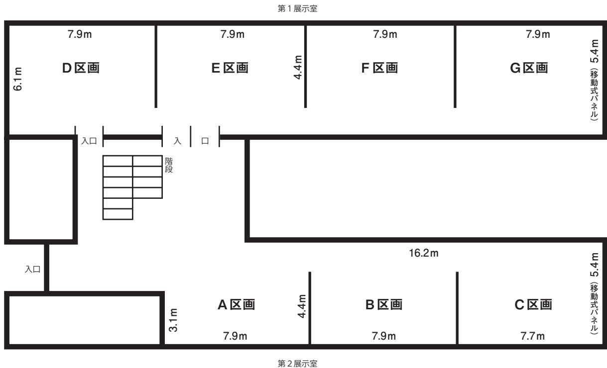
豊橋市民文化会館 2階 展示室図面
